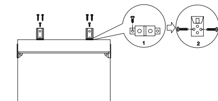
Рисунок 6 – Монтаж на стену
