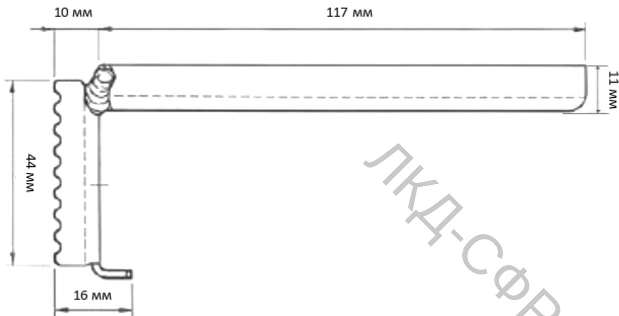
Вид сбоку
