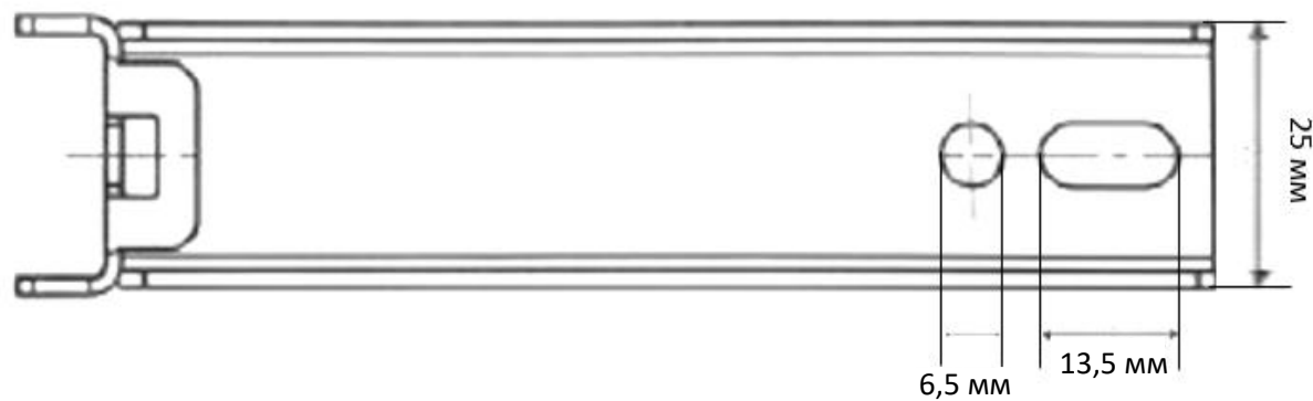
Вид снизу
