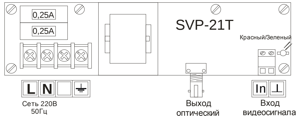
Рис. 1. Расположение разъемов и элементов индикации.
