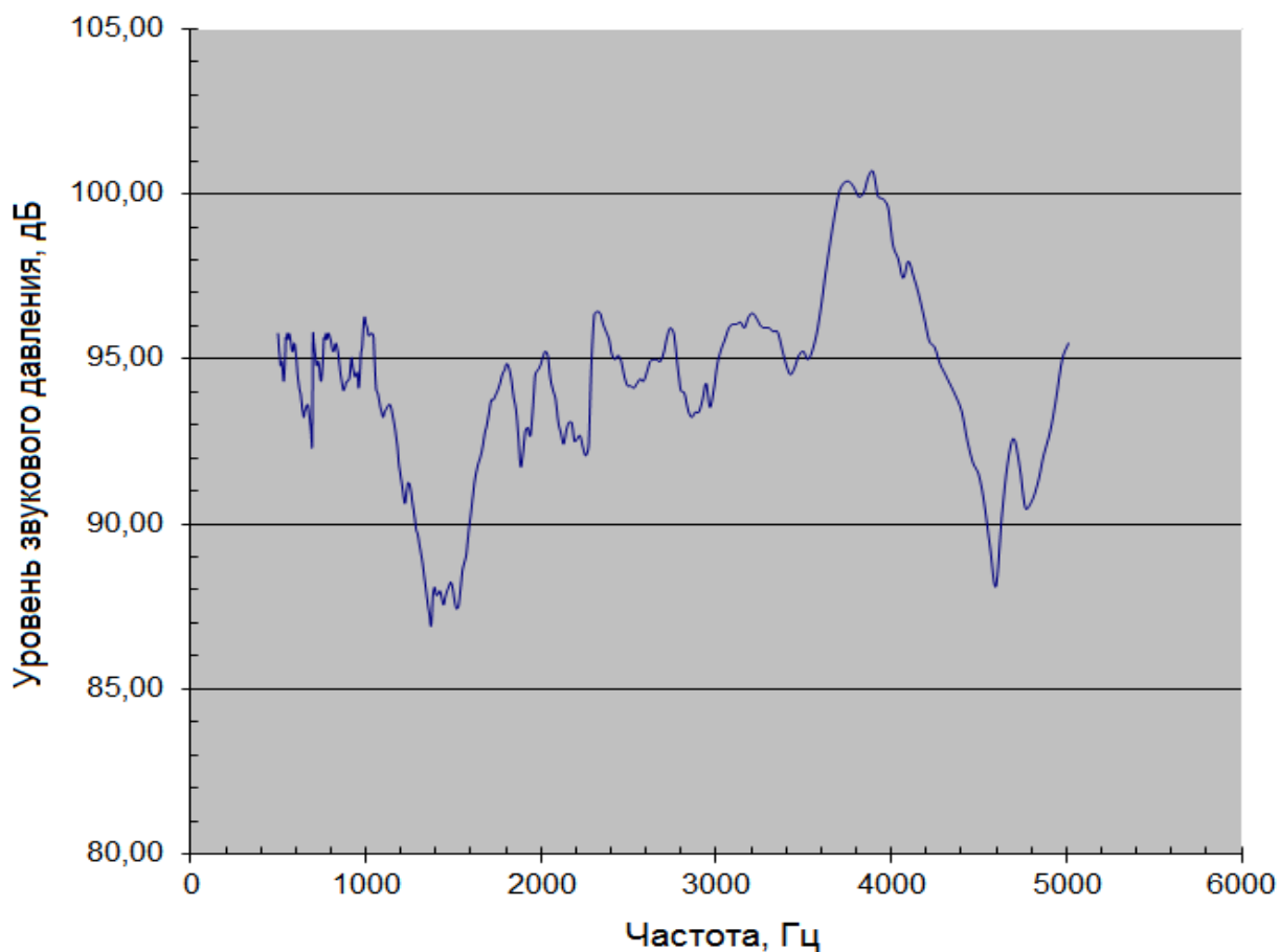
Рисунок 1 – Амплитудно-частотная характеристика оповещателя.
