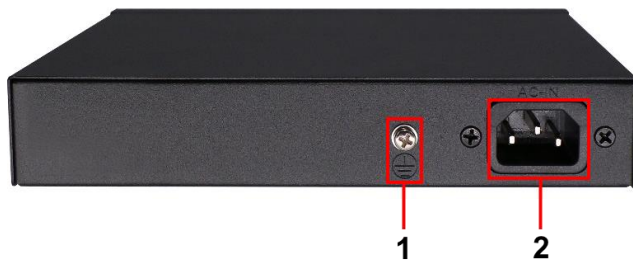
Рис. 3 Коммутатор SW-21000(120W), разъемы и клеммы на задней панели
