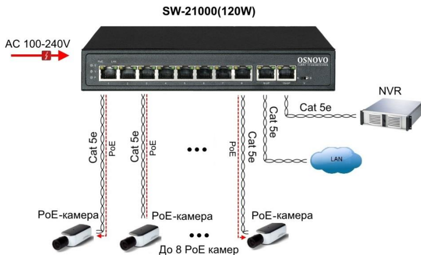
Рис.4 Типовая схема подключения коммутатора SW-21000(120W)
