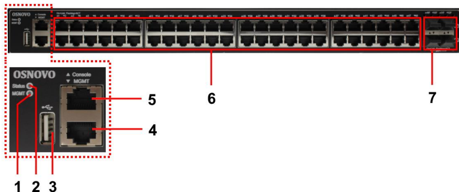
Рис.5 Коммутатор SW-48G4X-L3ST, разъемы, кнопки и индикаторы на передней панели
