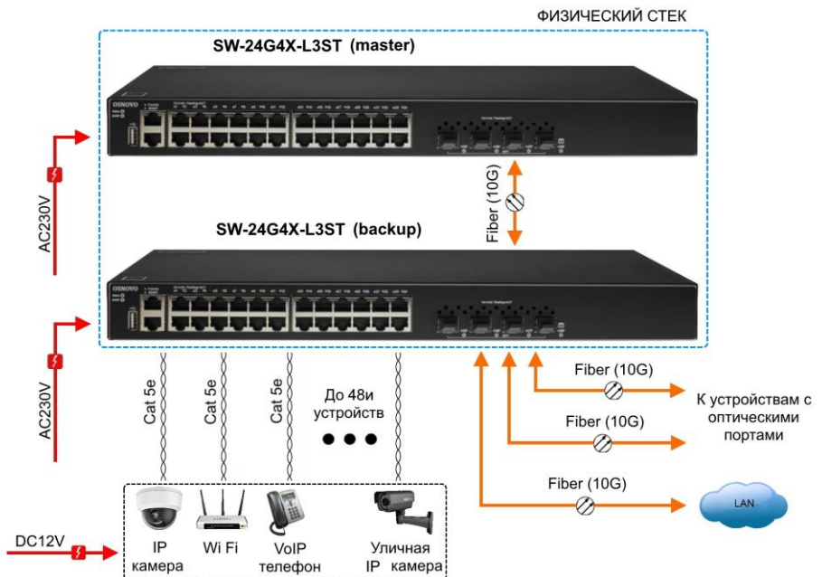
Рис.8 Стелевое подключение коммутаторов на примере SW-24G4X-L3ST.
