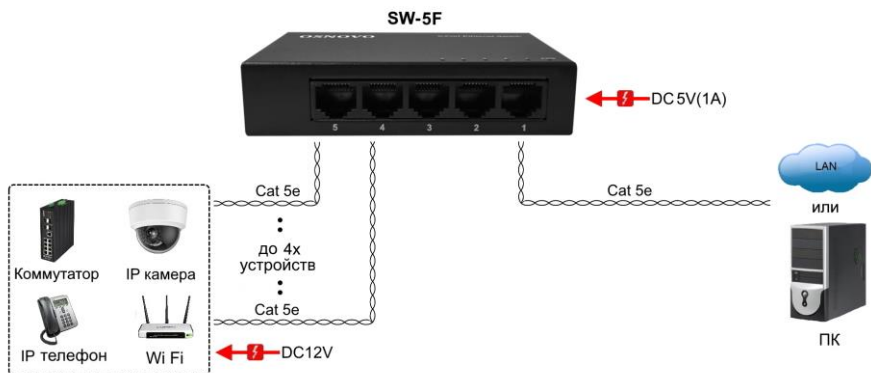
Рис.4 Типовая схема подключения коммутатора SW-5F.
