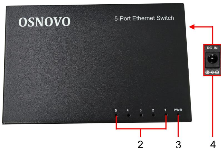
Рис.3 Коммутатор SW-5F, индикаторы и разъемы верхней и боковой панелей.
