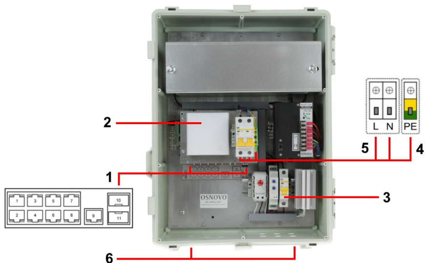
Рис.4 Подключение коммутатора SW-60812/WU
