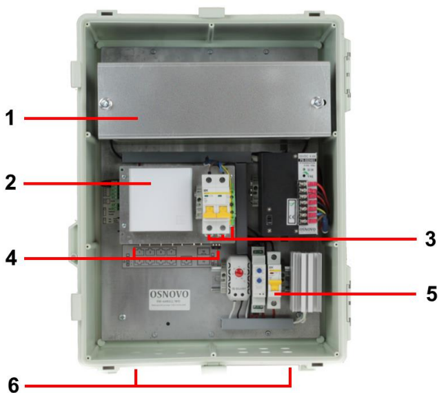
Рис.2 Коммутатор SW-60812/WU, вид внутри
