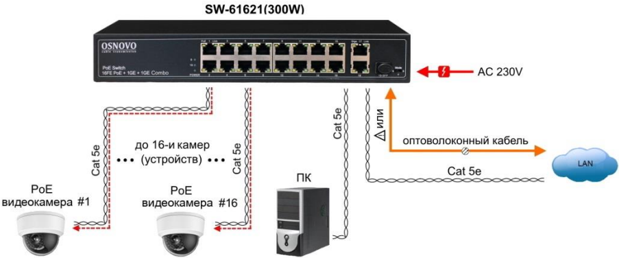
Рис.4 Типовая схема подключения коммутатора SW-61621(300W)
