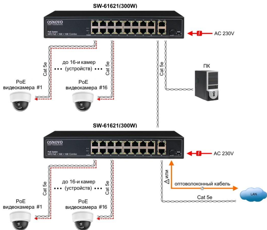
Рис.5 Схема каскадного подключения коммутатора SW-61621(300W)
