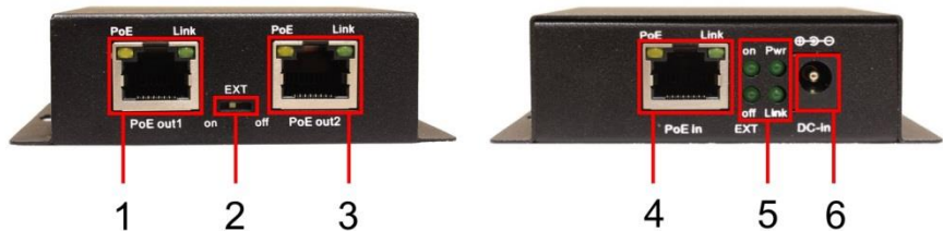
Рис. 3 Панели подключения коммутатора/удлинителя SW-8030/D(90W)
