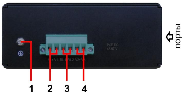
Рис.3 Коммутатор SW-80402-I(port60W, 240W), разъемы и переключатели верхней панели
