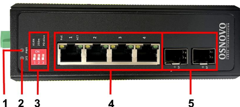
Рис.2 Коммутатор SW-80402-I(port60W, 240W), разъемы и индикаторы на передней панели
