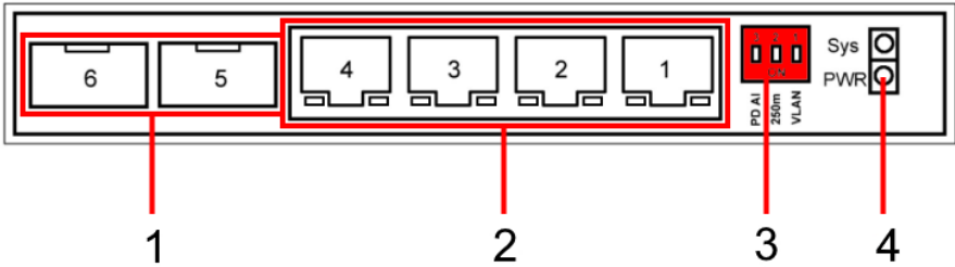
Рис.3 Коммутатор SW-80402-W(port 60W), разъемы и индикаторы
