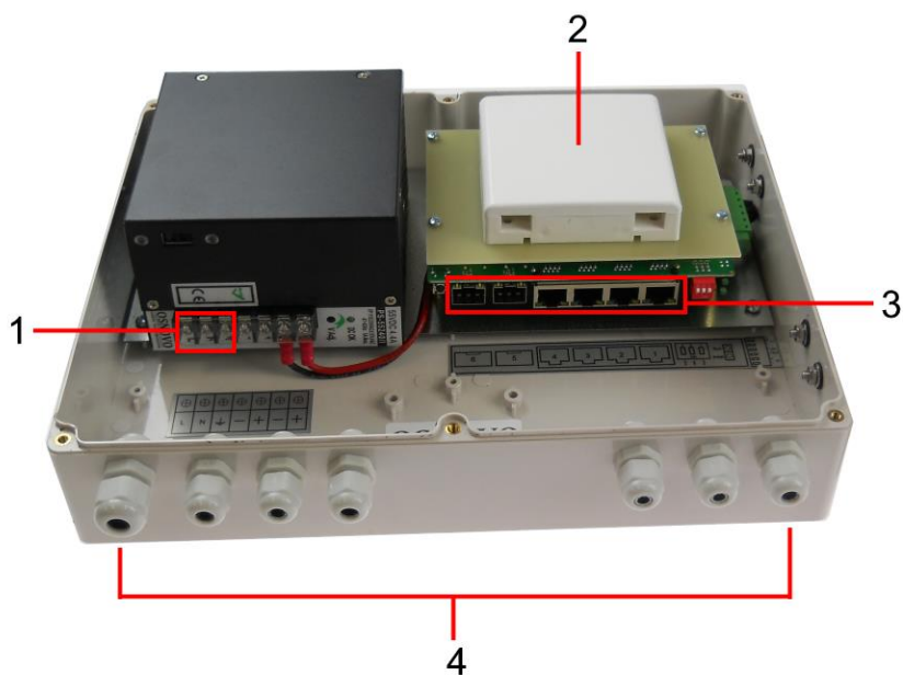
Рис.2 Коммутатор SW-80402-W(port 60W), вид внутри
