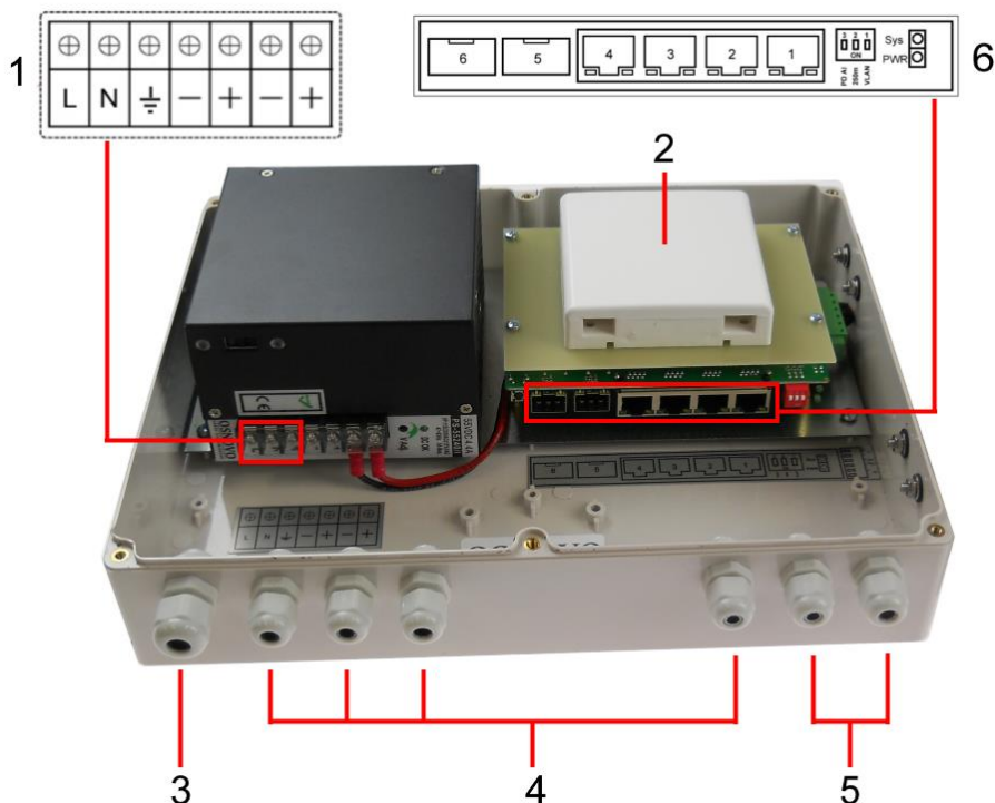
Рис.5 Подключение коммутатора SW-80402-W(port 60W)
