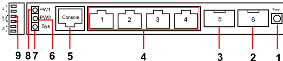
Рис.3 Уличный коммутатор SW-80402-WLU(port 90W), разъемы, кнопки и индикаторы
