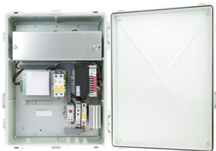
Рис. 2 Уличный коммутатор SW-80402-WLU(port 90W), вид внутри
