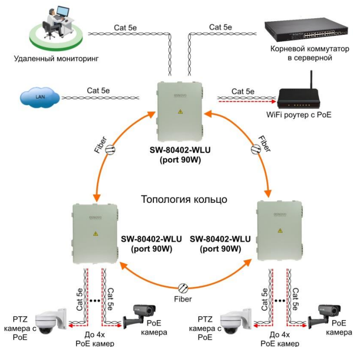
Рис. 7 Схема подключения уличного коммутатора SW-80402-WLU(port 90W) в топологии «кольцо»
