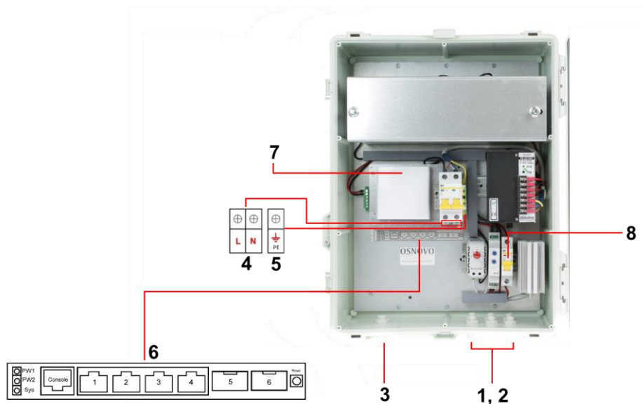
Рис. 4 Подключение уличного коммутатора SW-80402-WLU(port 90W) Подключение уличного коммутатора SW-80402-WLU(port 90W) осуществляются в следующей последовательности:
