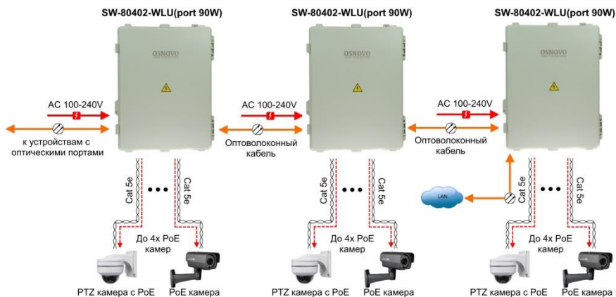
Рис. 6 Типовая схема подключения уличного коммутатора SW-80402-WLU(port 90W)
