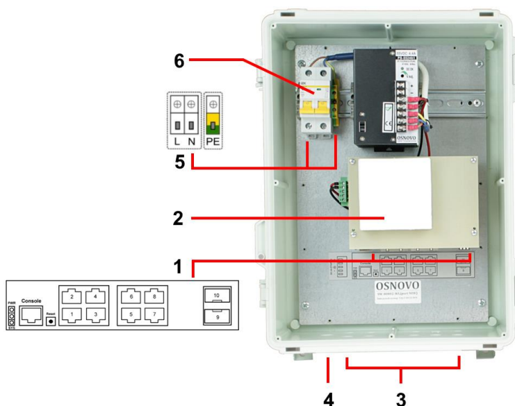
Рис. 4 Подключение уличного коммутатора SW-80802-WL(port 90W)
