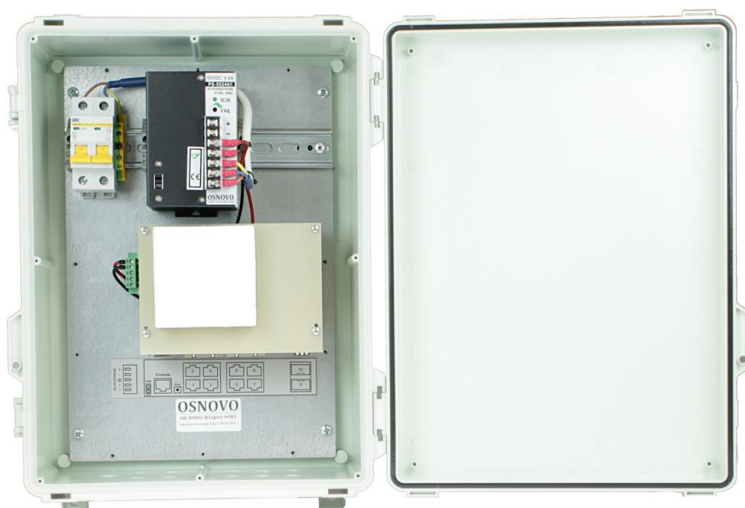
Рис. 2 Уличный коммутатор SW-80802-WL(port 90W), внешний вид внутри
