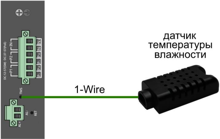
Рис.6 Схема подключения внешнего датчика температуры/влажности
