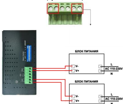
Рис.5 Схема подключения блоков питания к клеммной колодке коммутаторов SW-60822/ILR, SW-80822/ILR
