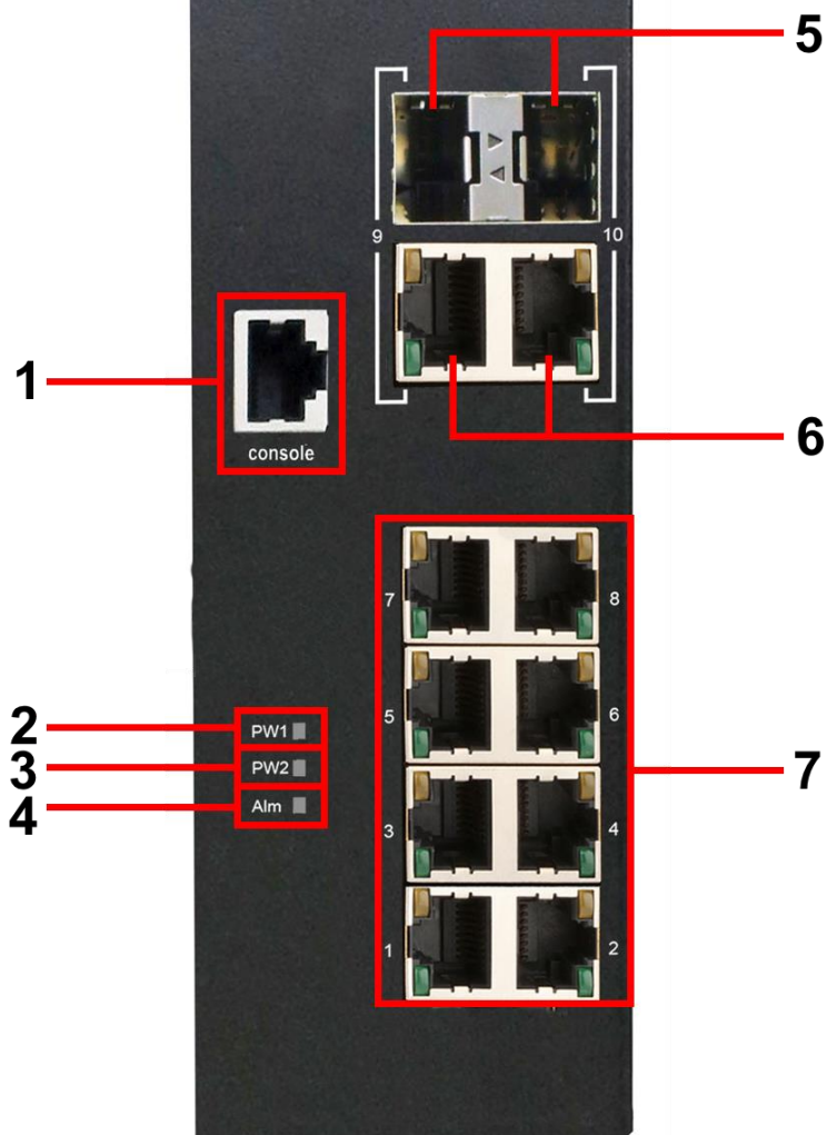
Рис. 2 Коммутаторы SW-60822/ILR (SW-80822/ILR), разъемы, кнопки и индикаторы передней панели
