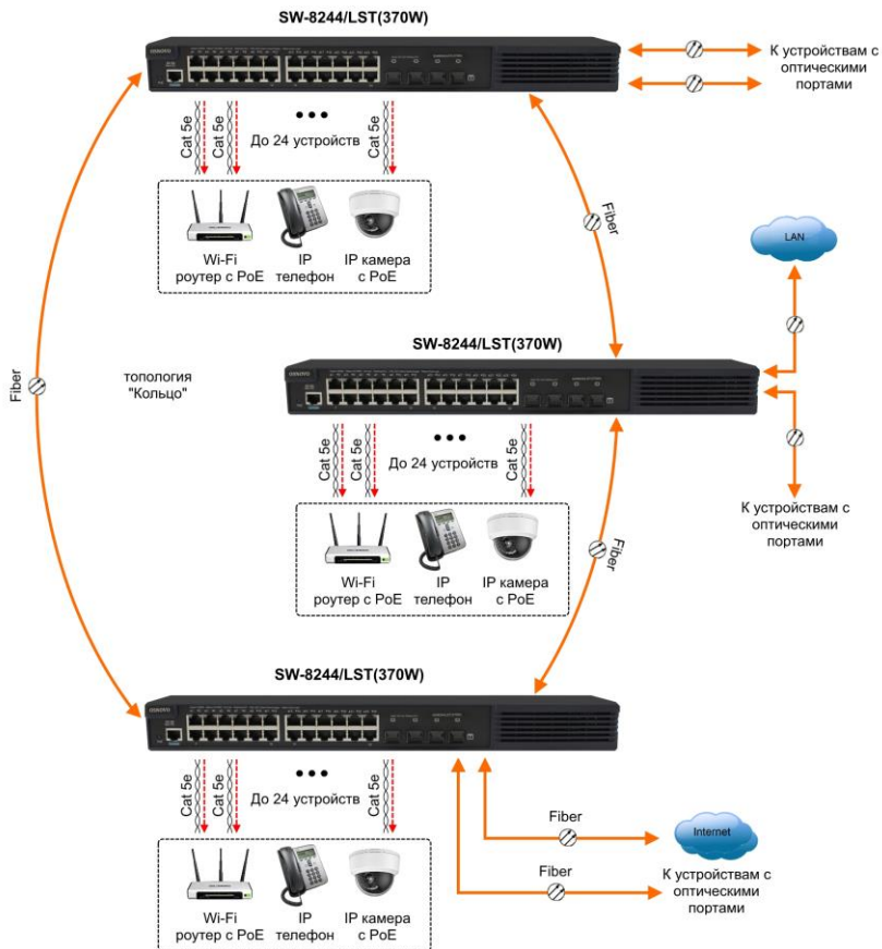
Рис.7 Схема подключения коммутатора SW-8244/LST(370W) при работе в кольцевой топологии
