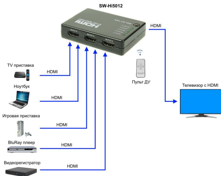
Рис.5 Типовая схема подключения HDMI коммутатора SW-Hi5012
