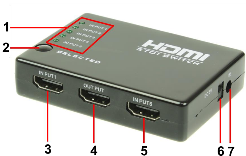
Рис.2 HDMI коммутатор SW-Hi5012, разъемы и индикаторы на передней панели
