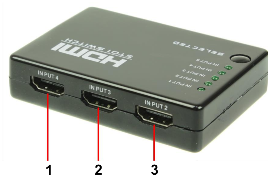
Рис.3 HDMI коммутатор SW-Hi5012, разъемы и индикаторы на задней панели
