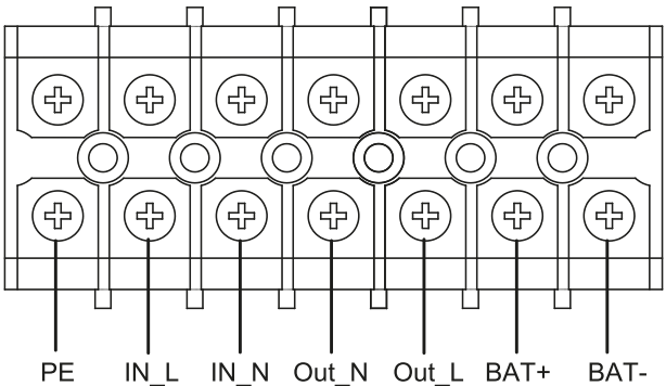
Рисунок 3. Клеммная колодка ИБП вариант подключения 1:1
