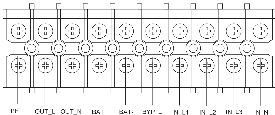
Рисунок 4. Клеммная колодка ИБП 10кВА вариант подключения 3:1
