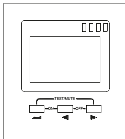
Рисунок 9. Панель управления
