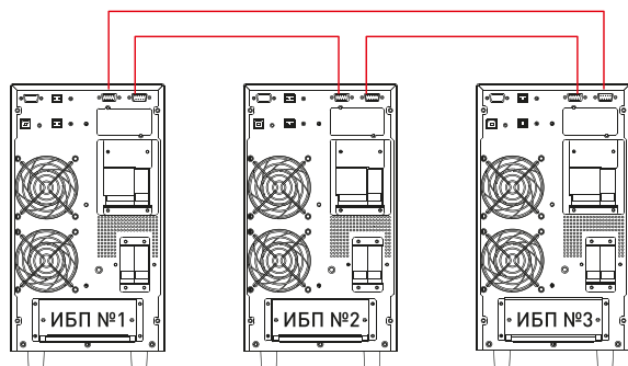
Рисунок 7. Подключение коммуникационных кабелей 3х ИБП
