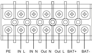
Рисунок 3. Клеммная колодка ИБП
