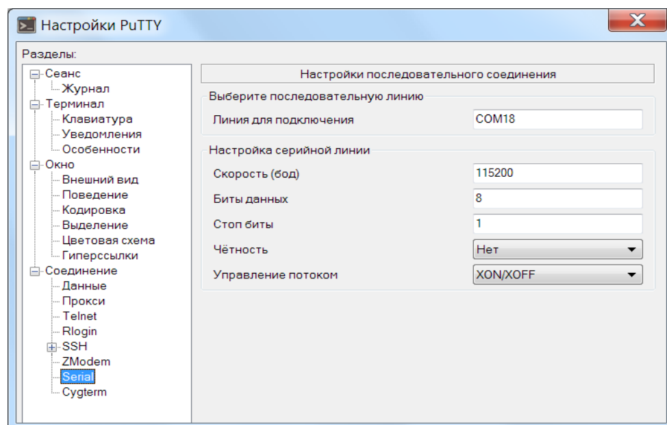
Рис. 5.5.2 — настройки соединения
