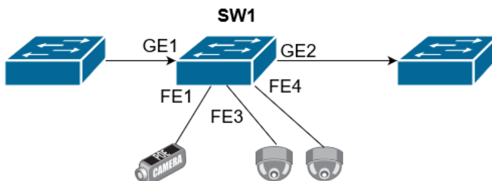
Рис. 5.3.18.2 Пример сети
