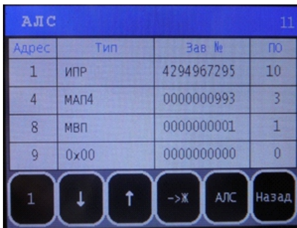
Рисунок 6 – Окно «АЛС»
