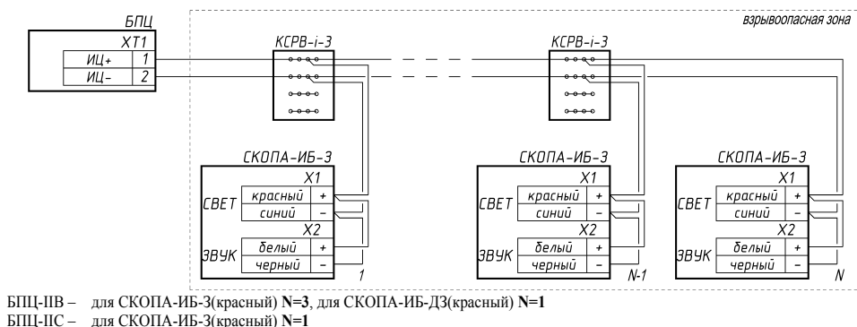
Рис. Б.3. Схема подключения оповещателей СКОПА-ИБ-З «ПОЖАР», СКОПА-ИБ-ДЗ «ПОЖАР» в один канал оповещения.
