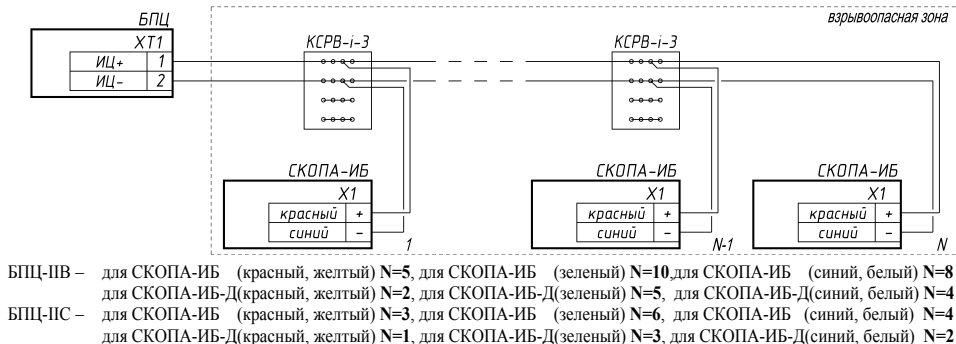
Рис. Б.1. Схема подключения оповещателей СКОПА-ИБ, СКОПА-ИБ-Д.
