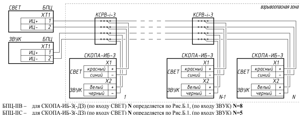
Рис. Б.2. Схема подключения оповещателей СКОПА-ИБ-З, СКОПА-ИБ-ДЗ с отдельными каналами оповещения: свет и звук.
