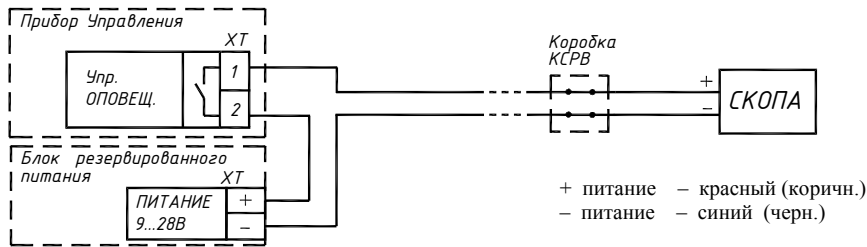
Рис. В.1. Схема подключения оповещателей СКОПА, СКОПА-С.
