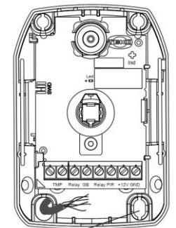
Заглушка отверстия для проводов
