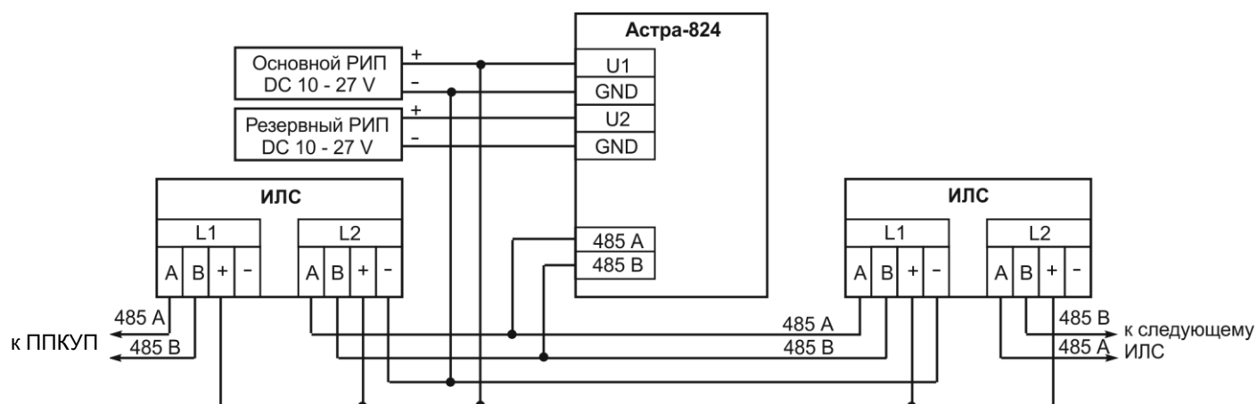
Рисунок 2 – Схема подключения изолятора «Астра-А ИЛС» к БРС «Астра-824»
