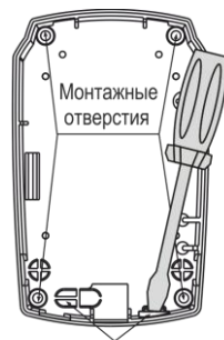
Отверстия для ввода проводов
