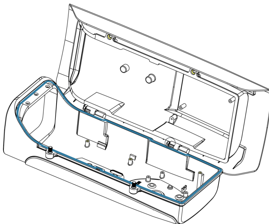
Рисунок 4.3 – Корпус
