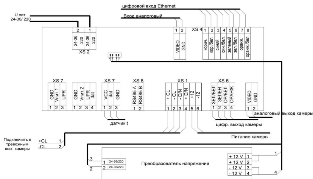
Рисунок 4.3 – Схема подключения термокожуха с напряжением питания 24–36 постоянного/переменного тока или 220 В переменного тока
