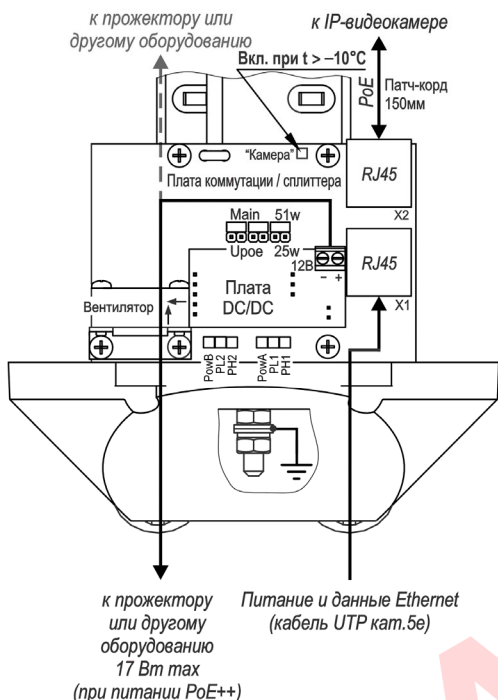
Рисунок 8 – Подключение ТГБ-7 TB-PoE++
