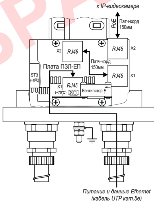
Рисунок 7 – Подключение ТГБ-4Г Ex IIC-PoE+ с платой ПЗЛ-ЕП
