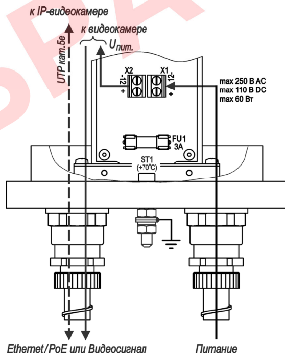
Рисунок 10 – Подключение ТГБ-4Г Ex IIC (без обогрева)
