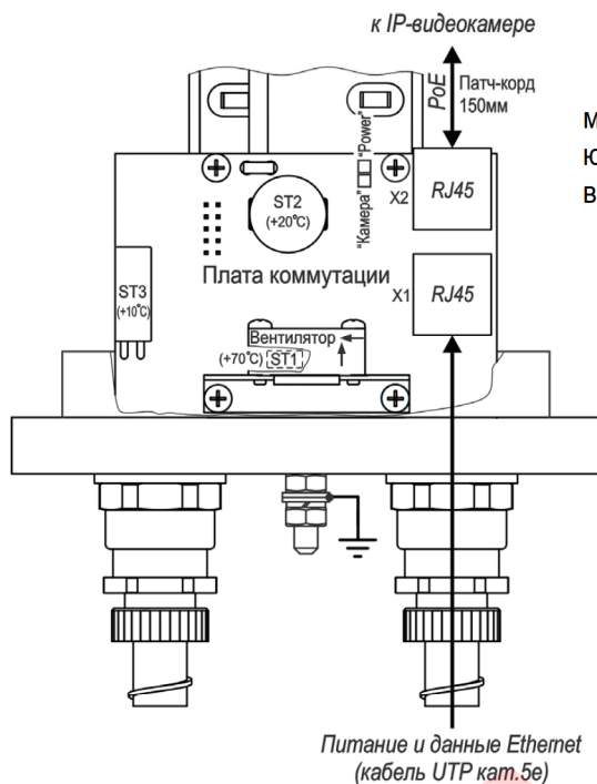
Рисунок 5 – Подключение ТГБ-4Г Ex IIC-PoE+
