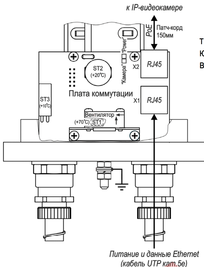
Рисунок 5 – Подключение ТГБ-4Г Ex IIC-PoE+
