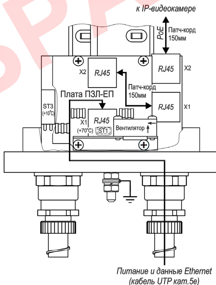
Рисунок 7 – Подключение ТГБ-4Г Ex IIC-PoE+ с платой ПЗЛ-ЕП
