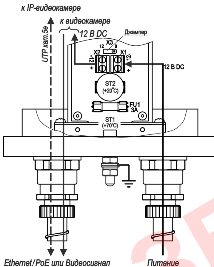
Рисунок 9 – Подключение ТГБ-4Г Ex IIC-12
