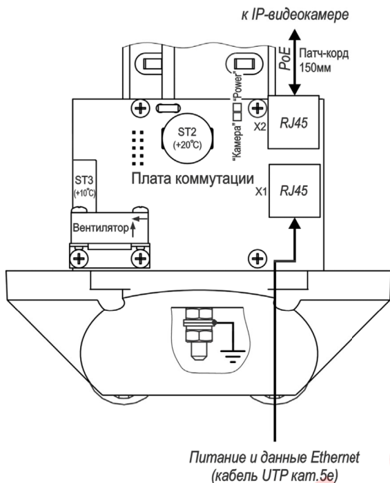
Рисунок 5 – Подключение ТГБ-7С-PoE+
