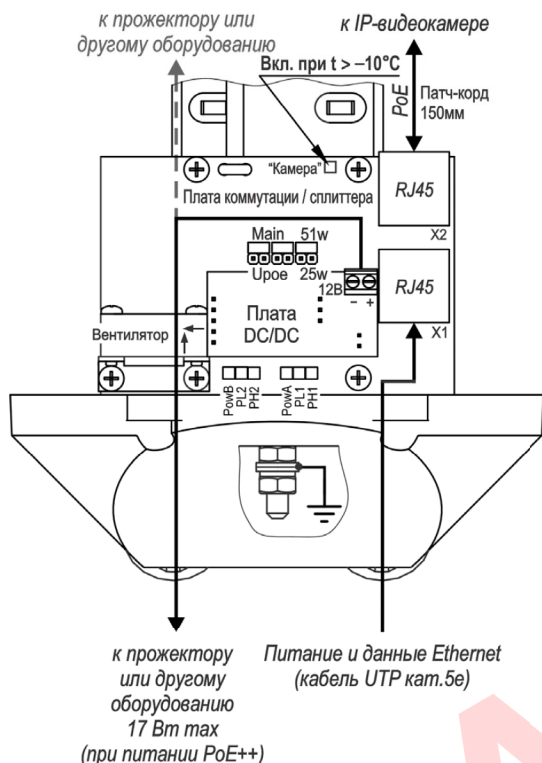
Рисунок 8 – Подключение ТГБ-7С-PoE++
