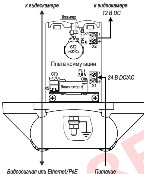
Рисунок 3 – Подключение ТГБ-7С-24/12
