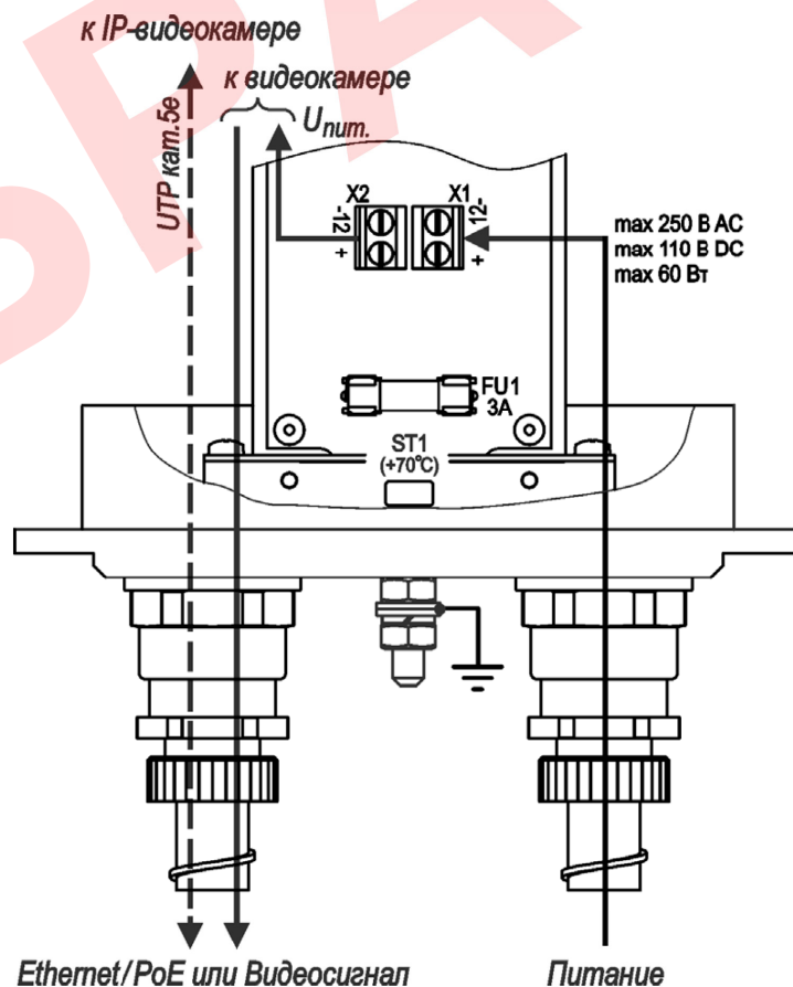
Рисунок 10 – Подключение ТГБ-8Г Ex (без обогрева)
