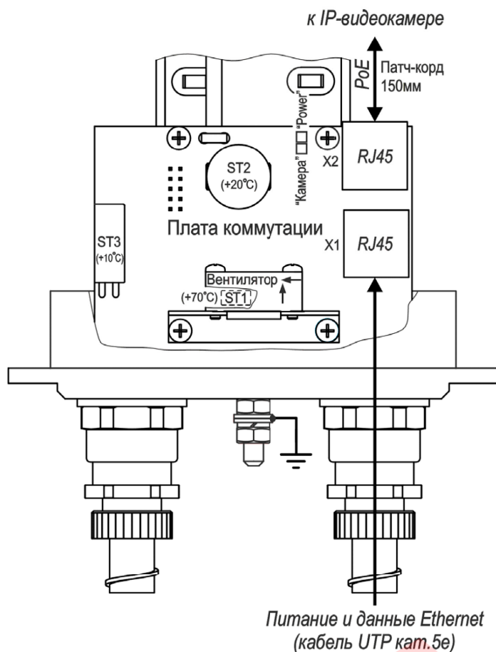
Рисунок 5 – Подключение ТГБ-8Г Ex-PoE+
