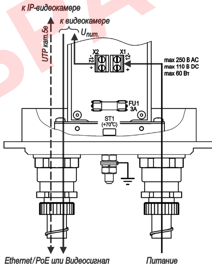
Рисунок 10 – Подключение ТГБ-8Г Ex (без обогрева)
