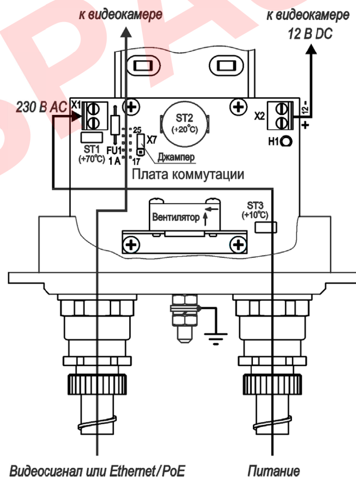
Рисунок 4 – Подключение ТГБ-8Г Ex-220/12
