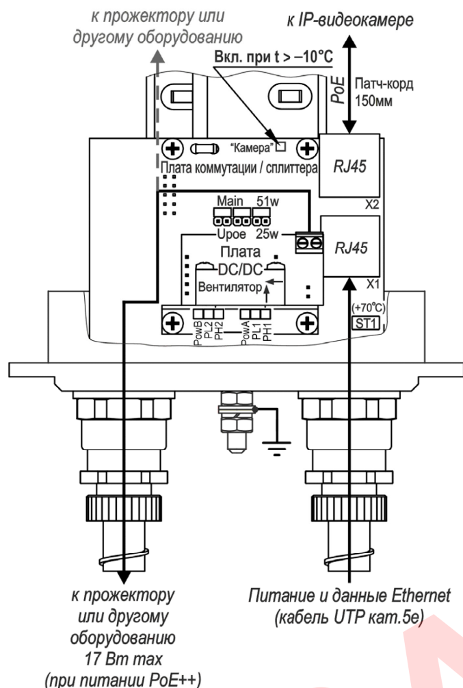
Рисунок 8 – Подключение ТГБ-8Г Ex-PoE++
