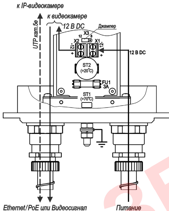
Рисунок 9 – Подключение ТГБ-8Г Ex-12
