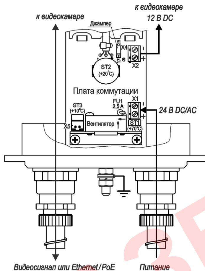
Рисунок 3 – Подключение ТГБ-8Г Ex-24/12
