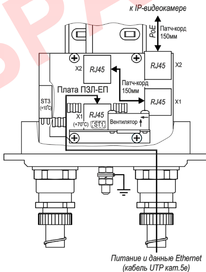
Рисунок 7 – Подключение ТГБ-8Г Ex-PoE+ с платой ПЗЛ-ЕП
