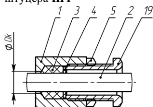
д) открытая прокладка кабеля в кабельном вводе КБО
