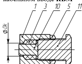
е) монтаж заглушки КГ
