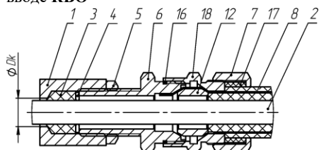
г) монтаж кабелем в металлорукаве в кабельном вводе КВМ
