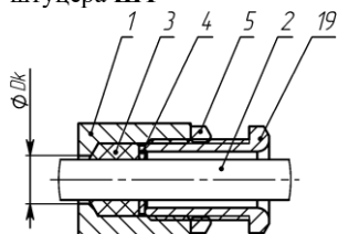
в) монтаж бронированным кабелем в кабельном вводе КВБ12
