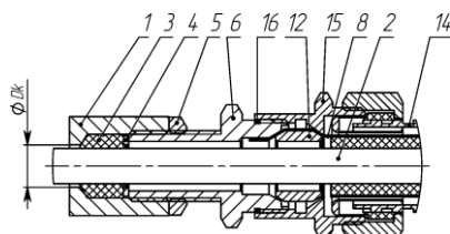
з) монтаж бронированным кабелем в металлорукаве в кабельном вводе КББМ
