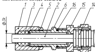
е) монтаж кабеля в металлорукаве в кабельном вводе КВМ
