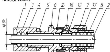
г) монтаж бронированным кабелем в кабельном вводе КВБ12
