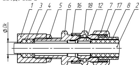
ж) монтаж бронированным кабелем в кабельном вводе КББУ
