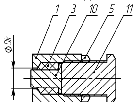
е) монтаж заглушки 3Г
