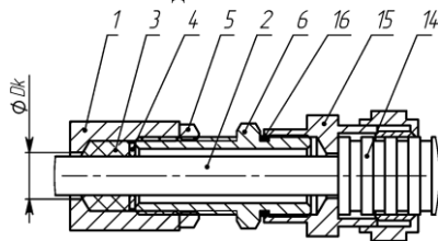
е) монтаж кабелем в металлорукаве в кабельном вводе КВМ
