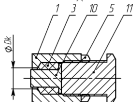
ж) монтаж заглушки ЗГ
