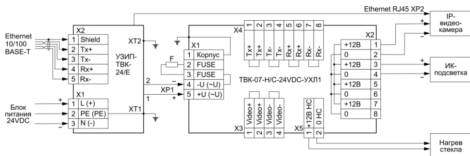
г) Подключение термокожуха на примере модификации ТБК-07-С-24VDC-YXL11 с устройством защиты УЗИП-TBK-24/E и IP-видеокамерой
