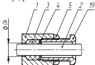
д) открытая прокладка кабеля в кабельном вводе КБО
