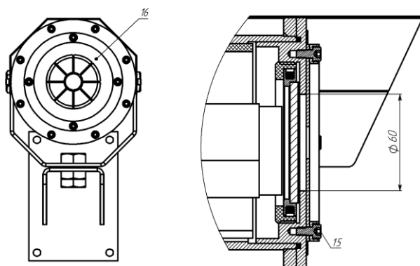
Рисунок 3. Внешний вид термокожуха ТВК-07-Н/С-“ВИЗОР” для тепловизора.
