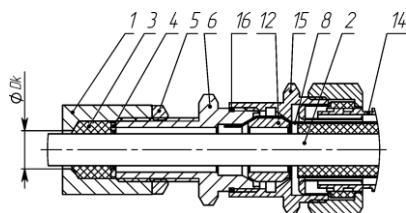
и) монтаж в трубной разводке с помощью штуцера ШТ
