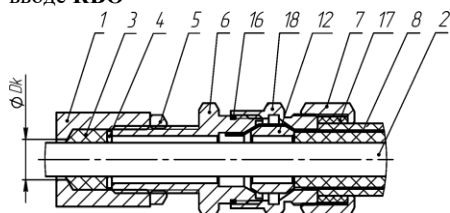
г) монтаж в трубной разводке с помощью штуцера ШТ
