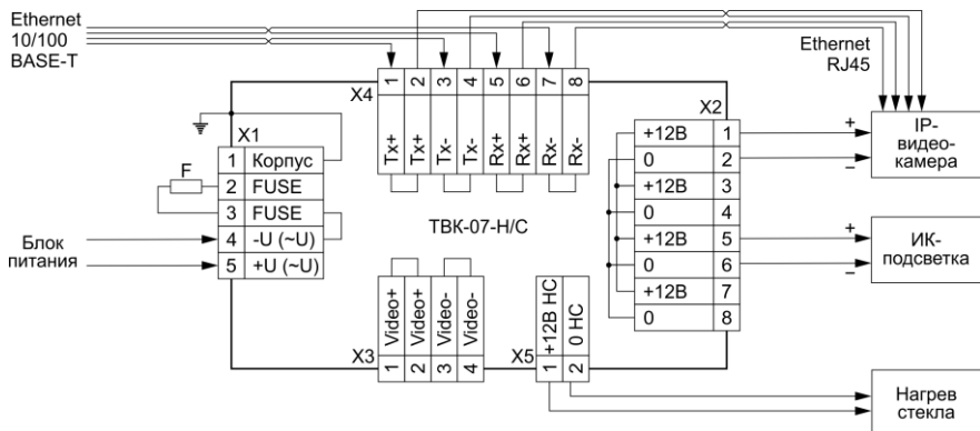
а) Подключение термокожуха на примере модификации ТБК-07-С-УХЛ1 с ИК-подсветкой и IP-видеокамерой
