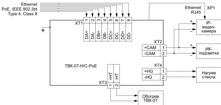
в) Подключение термокожуха на примере модификации ТВК-07-Н-PoE-УХЛ1 “АРКТИК” с ИК-подсветкой и IP-видеокамерой
