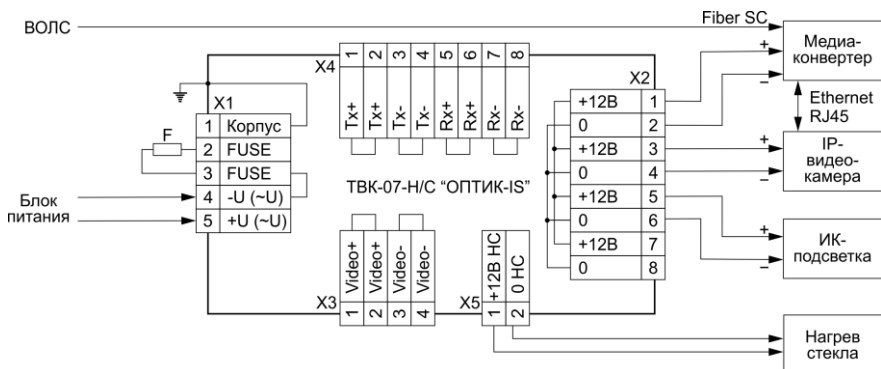
б) Подключение термокожуха на примере модификации ТВК-07-Н-“ОПТИК-IS”-УХЛ1 с ИК-подсветкой, IP-видеокамерой и медиаконвертером
